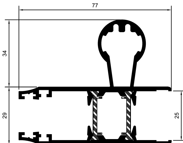
HOJA PERIMETRAL CON REFUERZO
