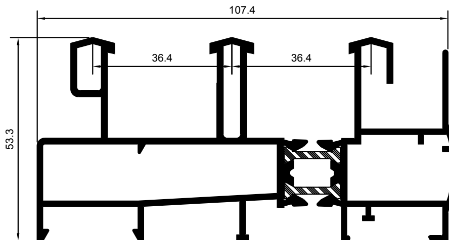
MARCO PERIMETRAL TRES CARRILES
