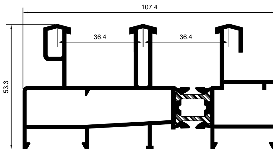
MARCO PERIMETRAL TRES CARRILES
