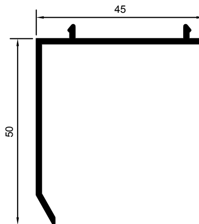
SOLAPE DE 50mm. PARA MARCOS ALIGERADOS
