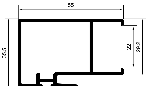
HOJA CENTRAL DOBLE ACRISTALAMIENTO
