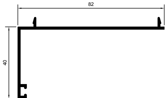
SOLAPE DE 40mm.
