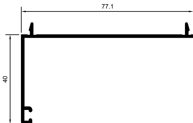
SOLAPE DE 40mm.
