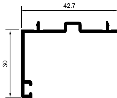
SOLAPE DE 30mm. PARA MARCOS ALIGERADOS
