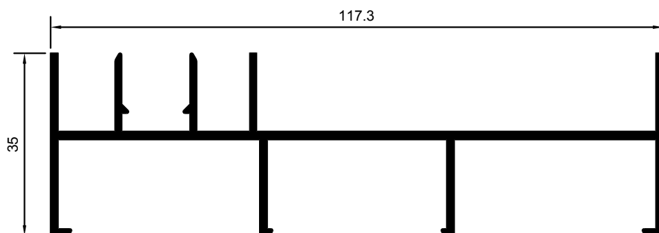
MARCO LATERAL TRES CARRILES
