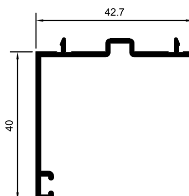
SOLAPE DE 40mm. PARA MARCOS ALIGERADOS
