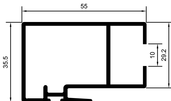
HOJA CENTRAL CRISTAL MONOLÍTICO
