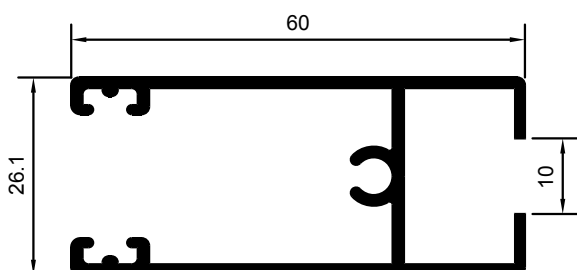
HOJA DE RUEDAS CRISTAL MONOLÍTICO
