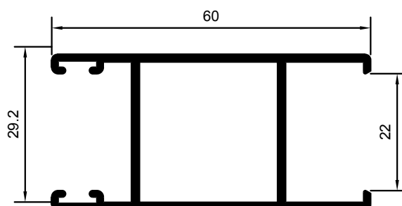
HOJA LATERAL DOBLE VIDRIO
