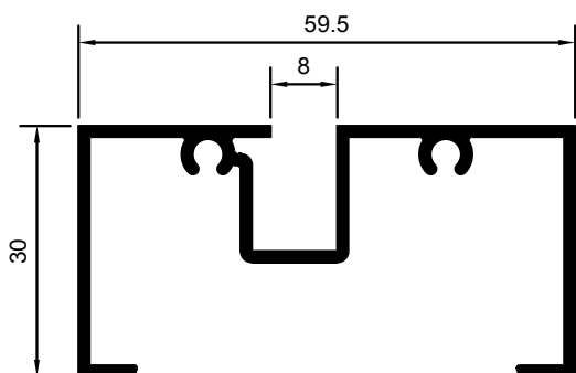
MARCO PARA FIJOS VIDRIO MONOLÍTICO M-2535
