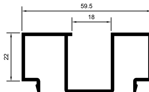
MARCO DE FIJOS DOBLE VIDRIO
