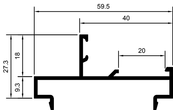
MARCO PARA FIJOS JUNQUILLO 40x20 CORTO
