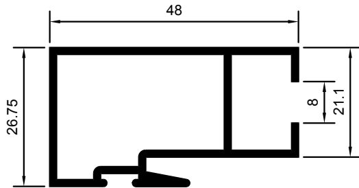
HOJA CENTRAL VIDRIO MONOLÍTICO
