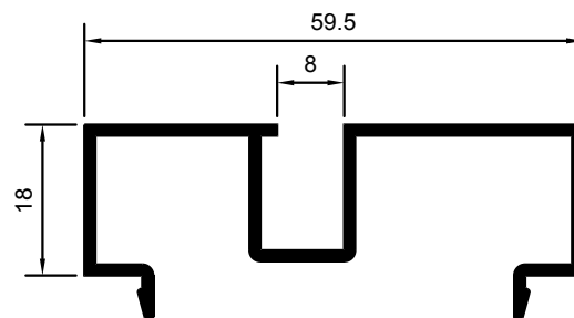
MARCO PARA FIJOS VIDRIO MONOLÍTICO
