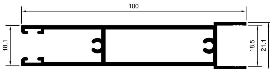
ZÓCALO DOBLE VIDRIO
