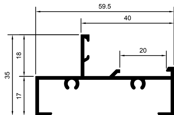
MARCO PARA FIJOS JUNQUILLO 40x20 CORTO
