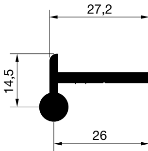
E-3603 Peso: 403 gr/m. P. Total: 96 mm.
