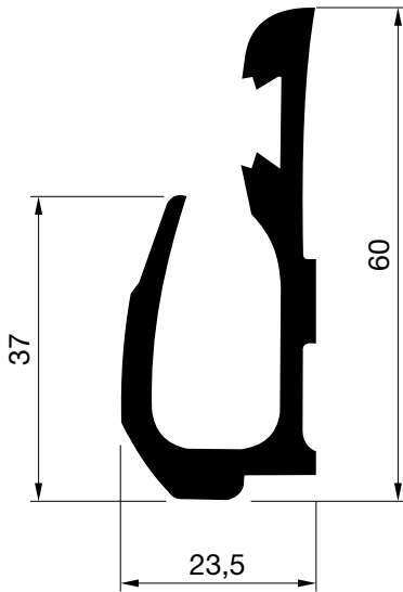
E-4754 Peso: 1105 gr/m. P. Total: 239 mm.
