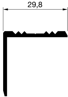
E-5675 Peso: 294 gr/m. P. Total: 123 mm.
