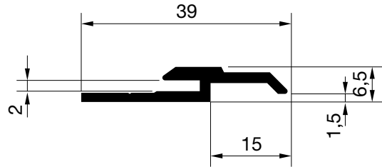
E-5273 Peso: 260 gr/m. P. Total: 102,3 mm.
