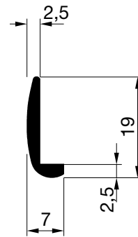
E - 5646 Peso: 126 gr/m. P. Total: 47 mm.
