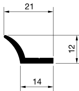
E-4232 Peso: 141 gr/m. P. Total: 57 mm.
