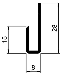
E-3775 Peso: 794 gr/m. P. Total: 98 mm.
