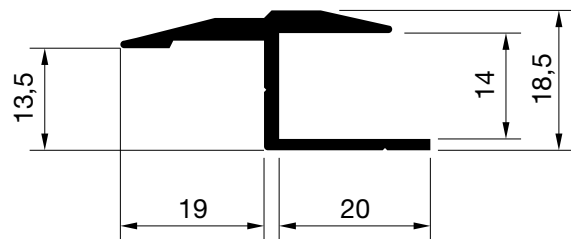
E-3601 Peso: 392 gr/m. P. Total: 146 mm.
