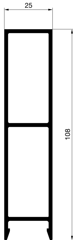
E-60063 Peso: 1423 gr/m. P. Total: 551 mm.
