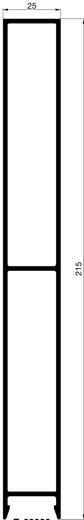
E-60022 Peso: 2355 gr/m. P. Total: 980 mm.
