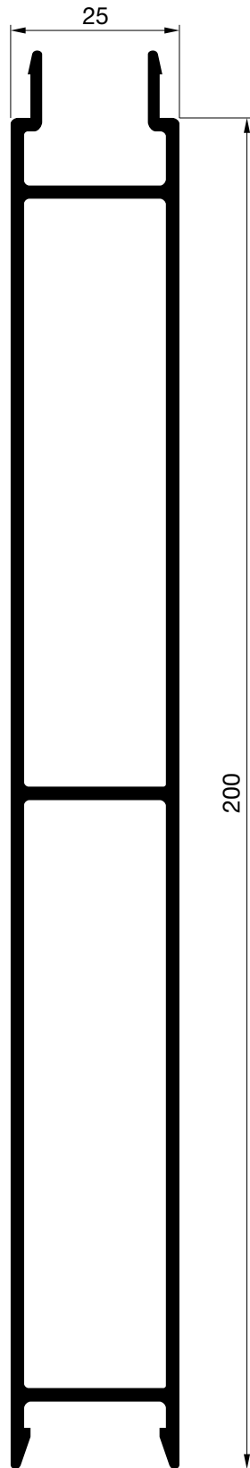
E-7505 Peso: 2686 gr/m. P. Total: 965 mm.
