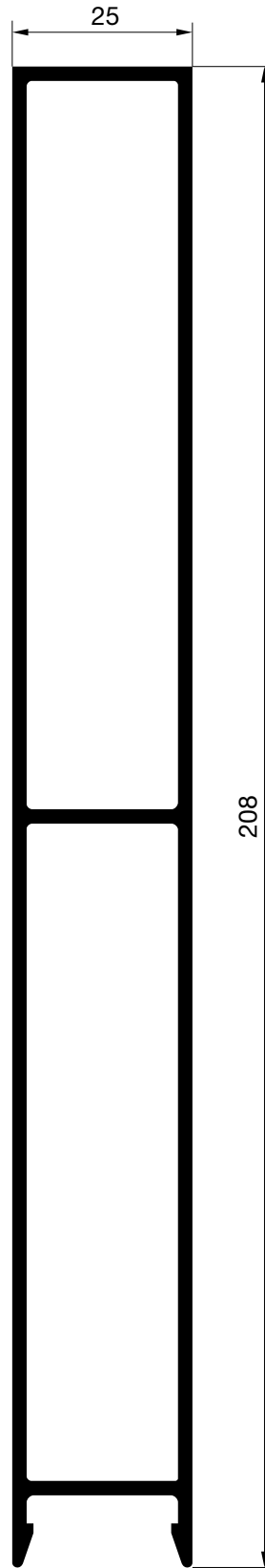
E-7504 Peso: 2395 gr/m. P. Total: 951 mm.
