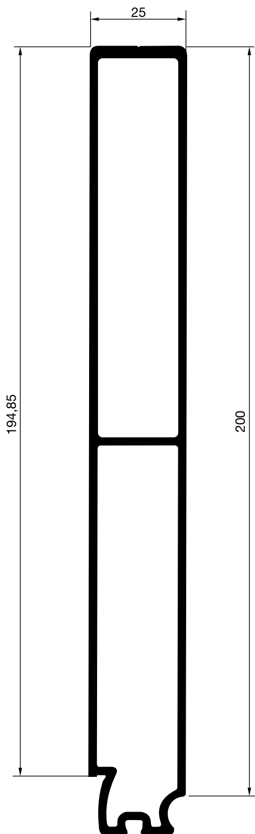
E-60102 Peso: 2360 gr/m. P. Total: 974 mm.
