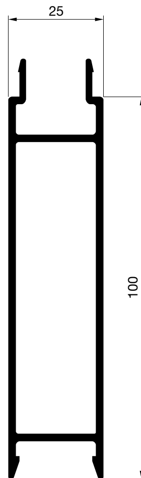
E-7684 Peso: 1365 gr/m. P. Total: 528 mm.
