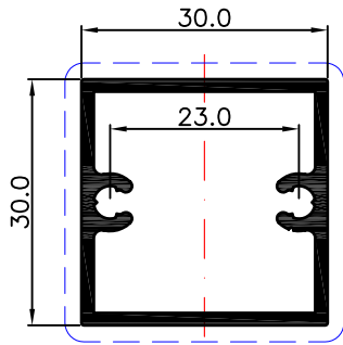
P00411 0.548 Kg/m 0.120 m 2 /m
