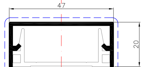
P03333 0.376 Kg/m 0.185 m 2 /m
