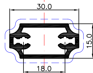
P53575 0.420 Kg/m 0.082 m 2 /m
