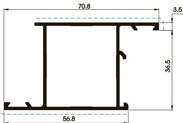
P02906 0,793 kg/m 0,266 m 2 /m
