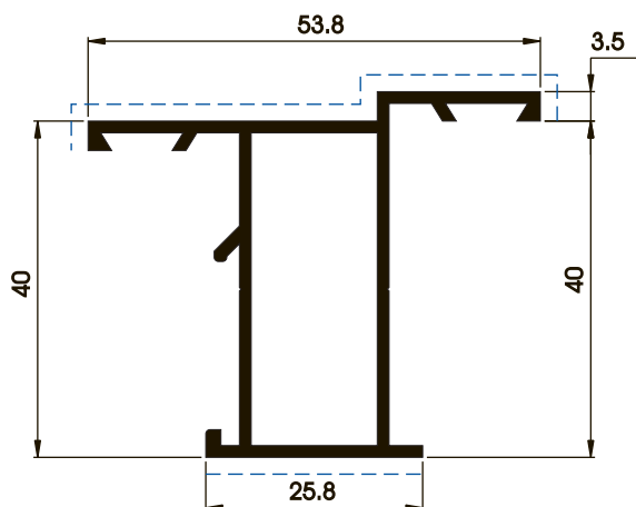
P01865 0,664 kg/m 0,243 m 2 /m
