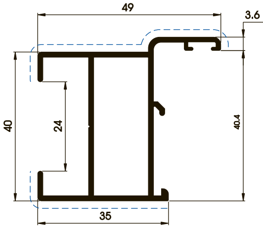
P04115 0,698 kg/m 0,267 m 2 /m
