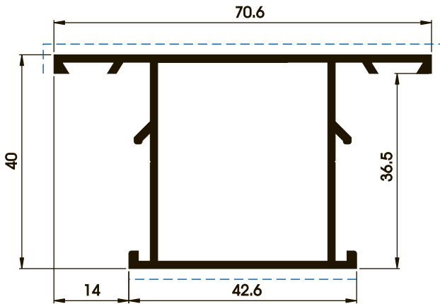
P01941 0,803 kg/m 0,286 m 2 /m
