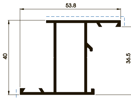
P01864 0,653 kg/m 0,236 m 2 /m
