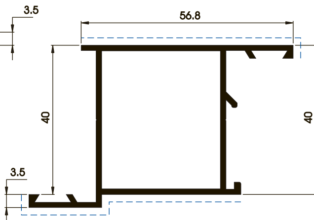
P01943 0,830 kg/m 0,277 m 2 /m
