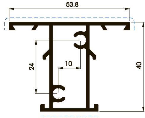
P01867 0,781 kg/m 0,247 m 2 /m
