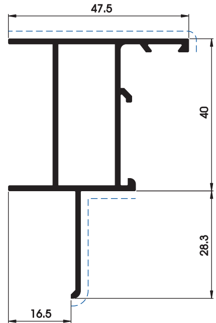
P01939 0,762 kg/m 0,285 m 2 /m
