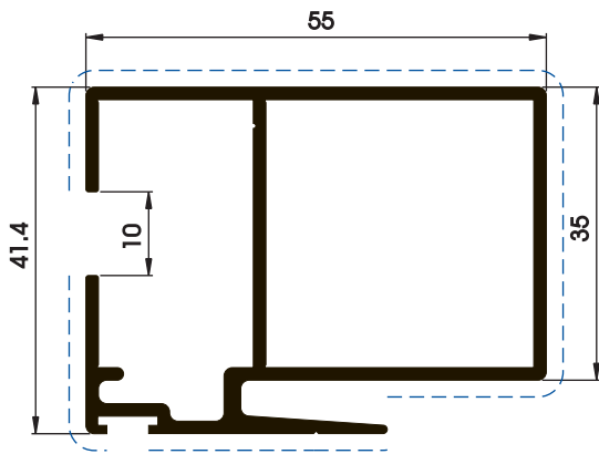
P03499 0,952 kg/m 0,332 m 2 /m
