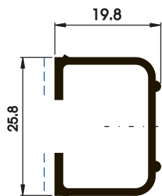
P04190 0,269 kg/m 0,147 m 2 /m
