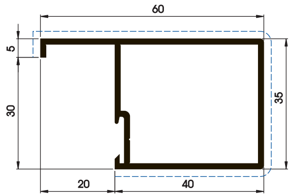
P03079 0,700 kg/m 0,208 m 2 /m
