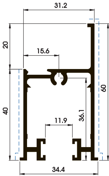
P03082 0,785 kg/m 0,376 m 2 /m
