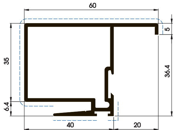
P03243 0,854 kg/m 0,276 m 2 /m
