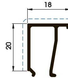
P03085 0,210 kg/m 0,128 m 2 /m
