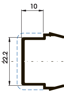
P03871 0,207 kg/m 0,127 m 2 /m
