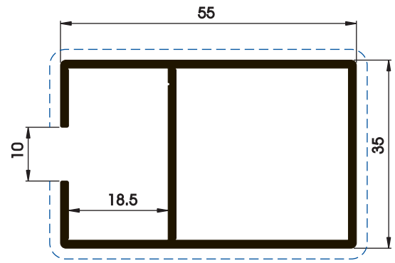
P03497 0,791 kg/m 0,263 m 2 /m
