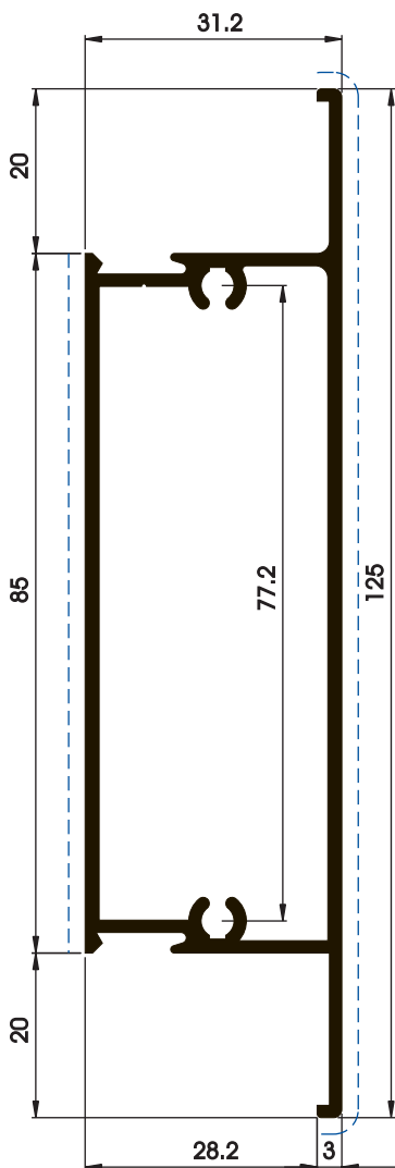
P03083 1,300 kg/m 0,333 m 2 /m
