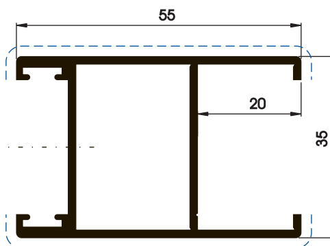
P03870 0,803 kg/m 0,271 m 2 /m
