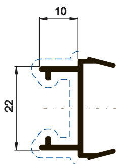
P04180 0,251 kg/m 0,140 m 2 /m
