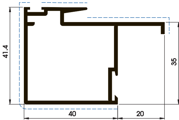
P03080 0,815 kg/m 0,248 m 2 /m
