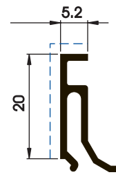
P03086 0,165 kg/m 0,102 m 2 /m
