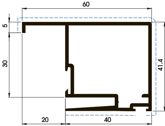
P03081 0,876 kg/m 0,274 m 2 /m
