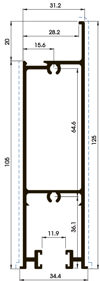
P03084 1,570 kg/m 0,504 m 2 /m
