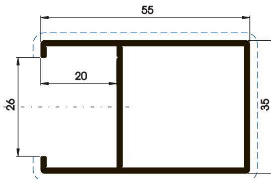
P03268 0,727 kg/m 0,232 m 2 /m
