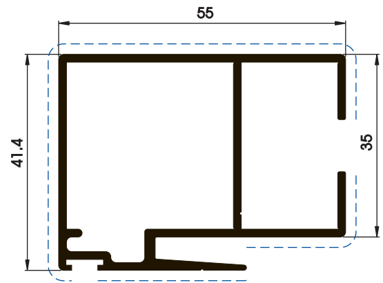
P03498 0,950 kg/m 0,317 m 2 /m
