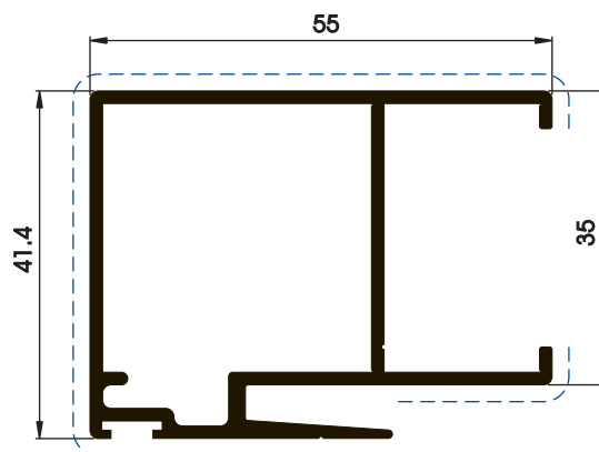
P03269 0,884 kg/m 0,283 m 2 /m
