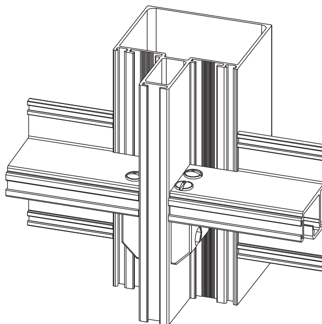
CONJUNTO ARMADO
