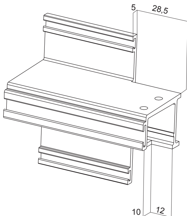
ENCASTRE PERFIL ADR-1437
