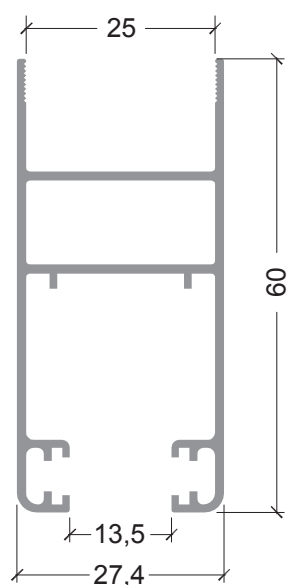
ADR 2744 0,653 kg/m
