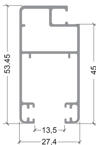
ADR 2740 0,659 kg/m
