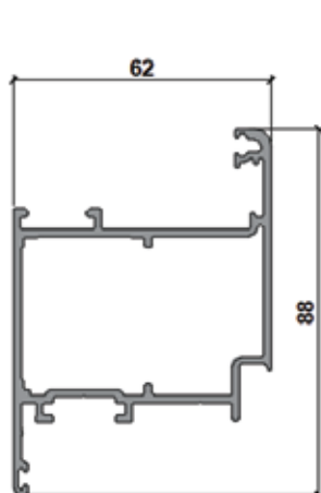
ADR 1475 Hoja Puerta Interior Peso: 1,498 kg/m
