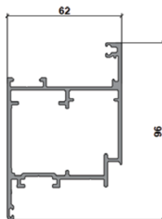
ADR 3706 Hoja Puerta XL Apertura Interior Peso: 1,718 kg/m
