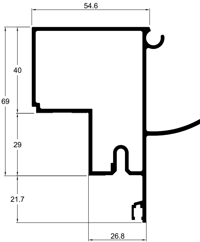
VL035 1,637 kg/m Coluna articulável com 69 mm
