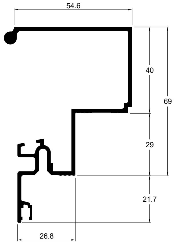
VL036 1,280 kg/m Coluna articulável com 69 mm
