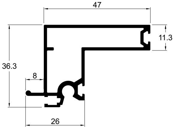
VL116 0,755 kg/m Montante/ travessa da folha
