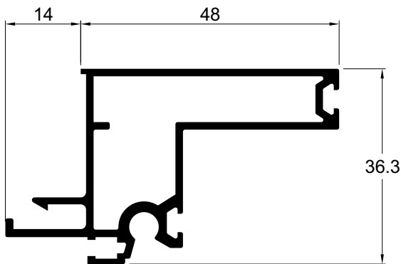
VL054 0,833 kg/m Montante / travessa da folha com bagueete
