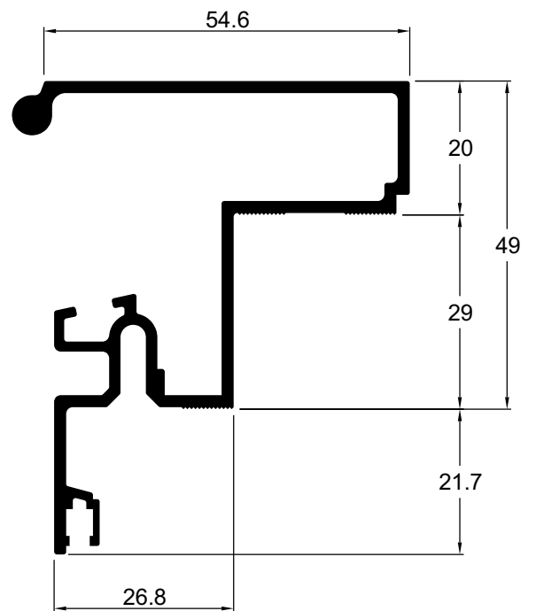
VL038 1,182 kg/m Coluna articulável com 49 mm
