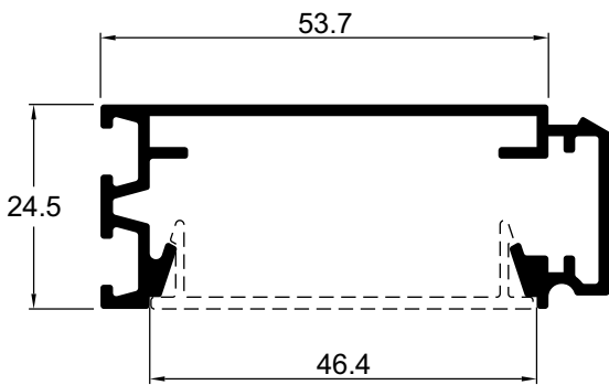
VL039 0,658 kg/m Arremate de folha
