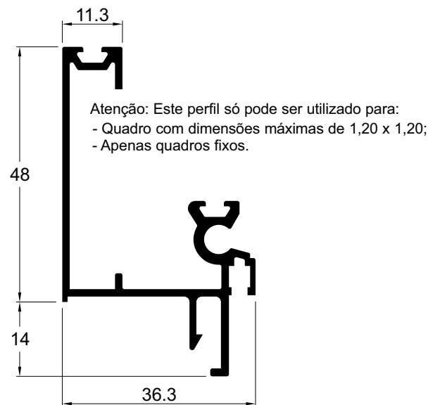
VL059 0,699 kg/m Montante da folha fixa com bagueete
