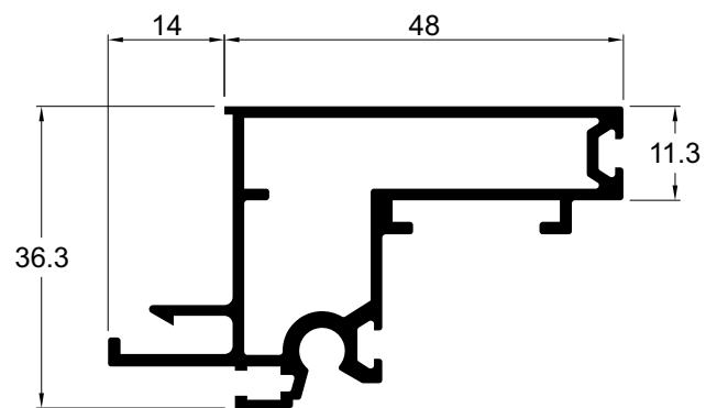
VL096 0,882 kg/m Travessa da folha maxim-ar com bagueete
