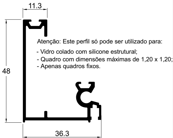
VL005 0,583 kg/m Montante / travessa da folha fixa
