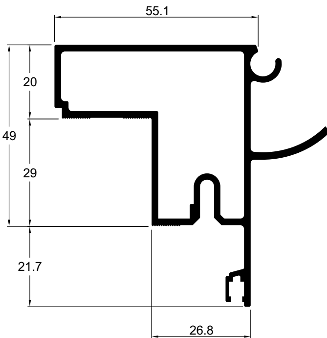
VL037 1,422 kg/m Coluna articulável com 49 mm
