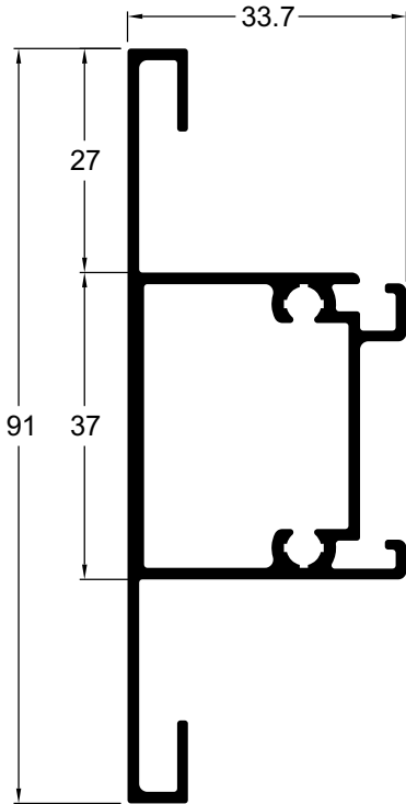
GN065 0,506 kg/m Baguete: vidro 24 mm Travessa porta de giro
