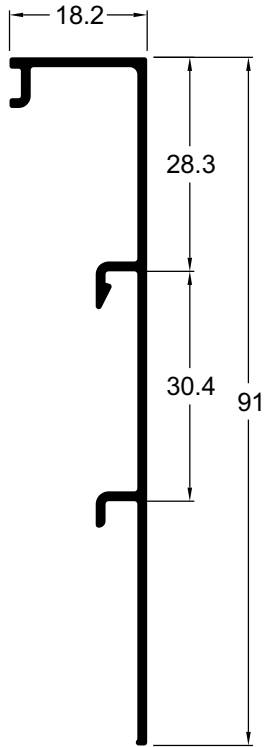
GN068 0,471 kg/m Baguete: vidro 4 a 6 mm Uso com vidro e Lambril Travessa porta de giro
