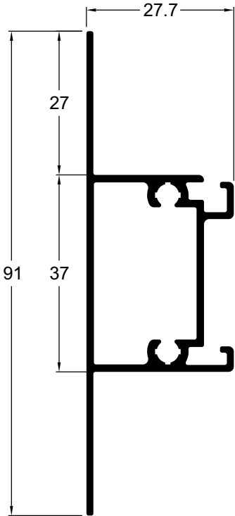
GN063 0,555 kg/m Baguete: vidro 4 a 6 mm Travessa porta de giro
