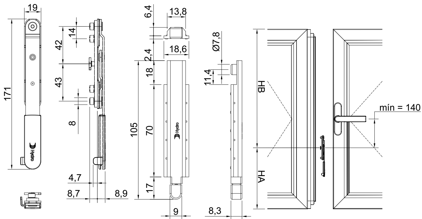
Limitador de Fecho # Closing limiter
