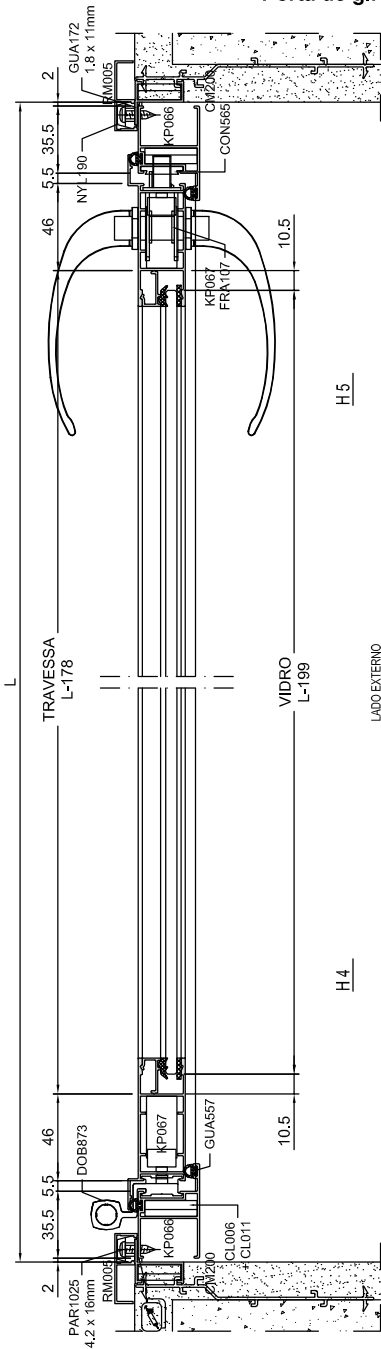
Porta de giro 1 folha
