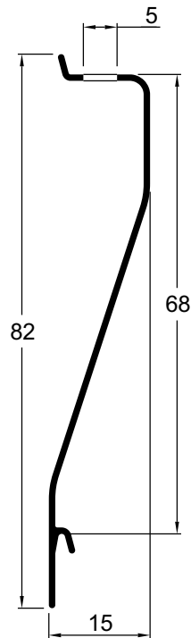
US621 0,259 kg/m Palheta veneziana ventilada
