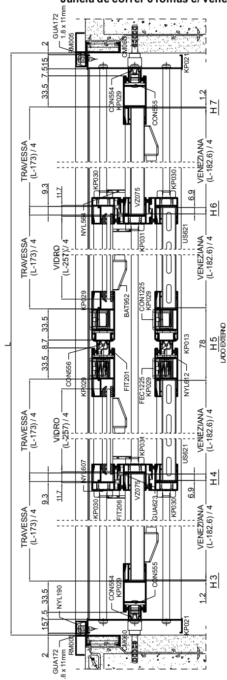
Janela de correr 6 folhas c/ venezianas
