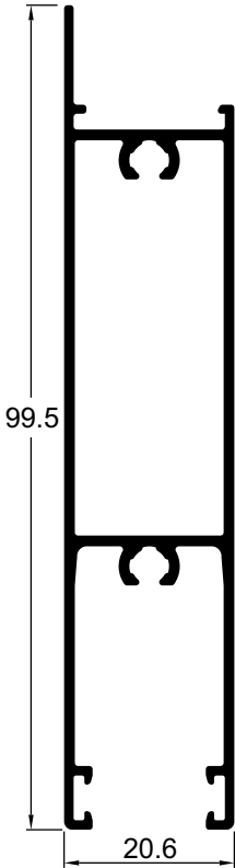
KP037 0,910 kg/m Folha travessa inferior (porta)
