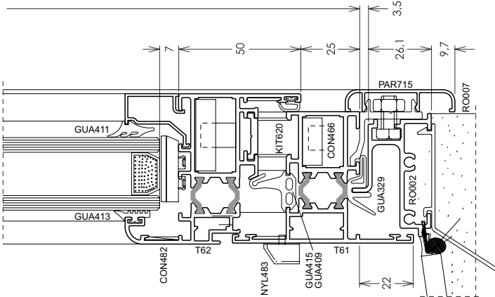
CORTE 01
