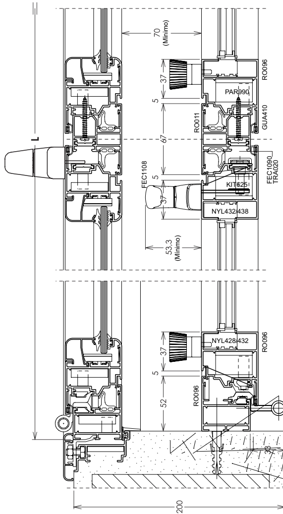
CORTE 04
