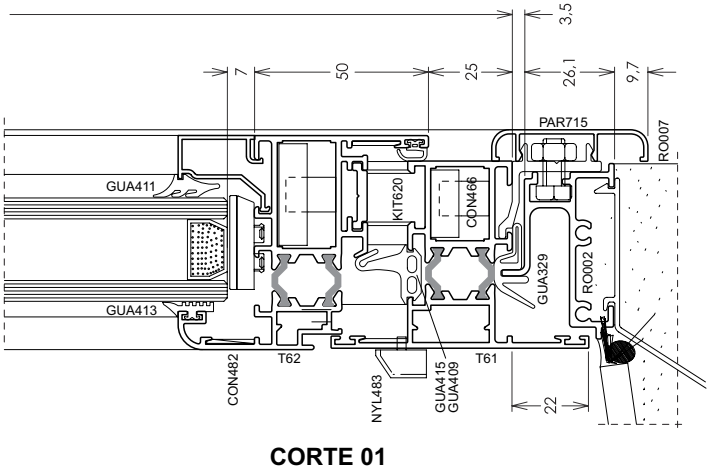
LADO EXTERNO
