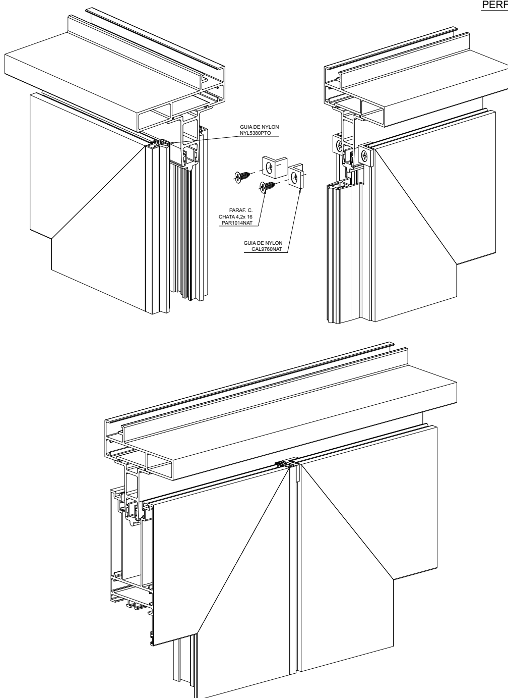
PERFIL - RO224
