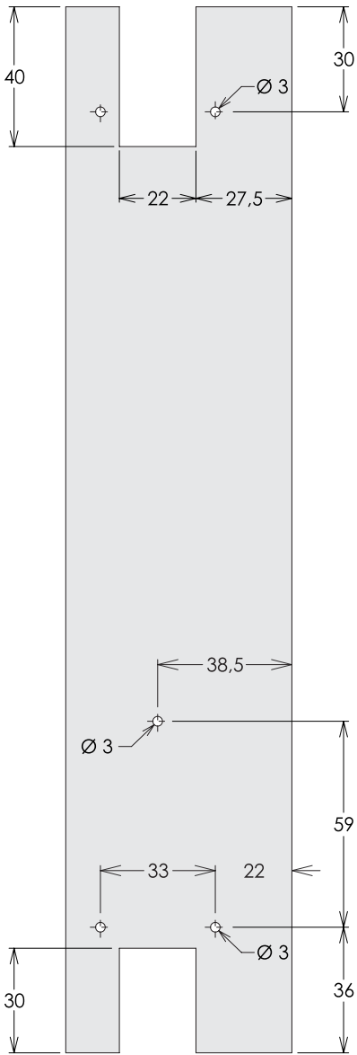
Lado Inferior
