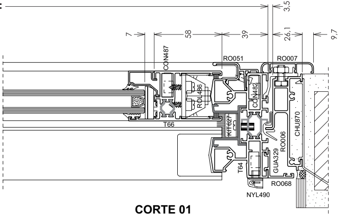
LADO EXTERNO
