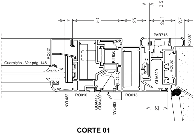
CORTE 01
