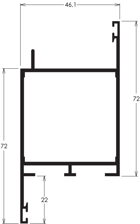
RO042 1,180 kg/m Folha travessa e montante
