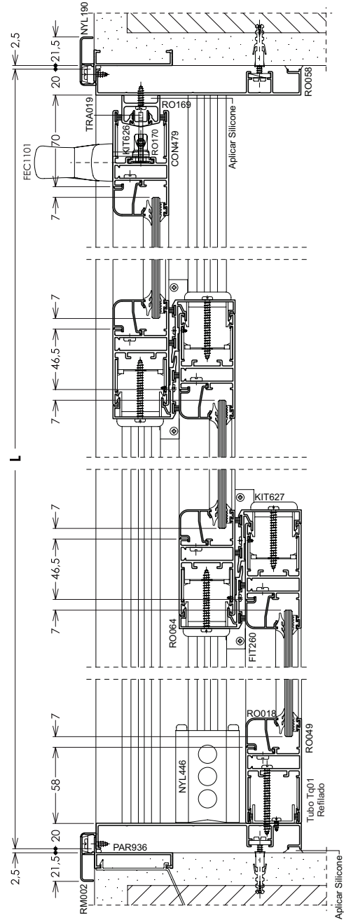
CORTE 06
