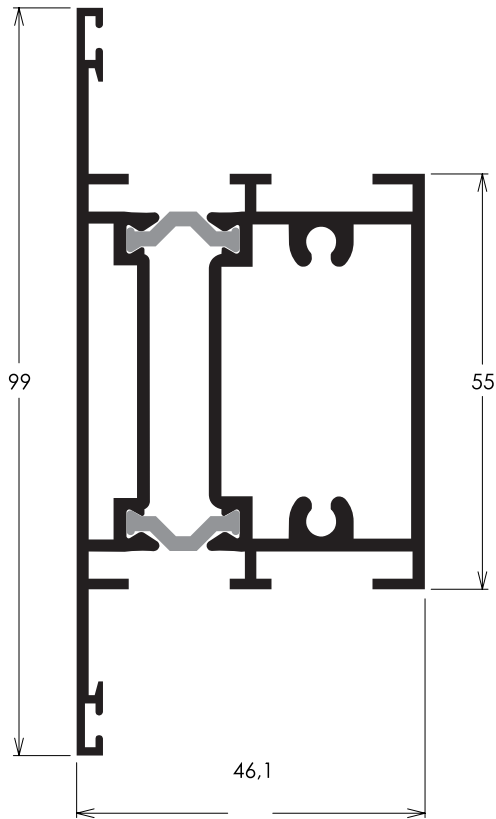
T77 Travessa intermediária
