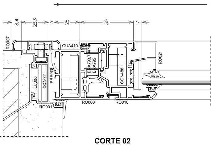
CORTE 02
