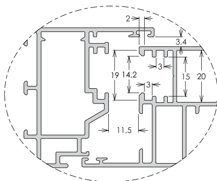
Detalhe B
