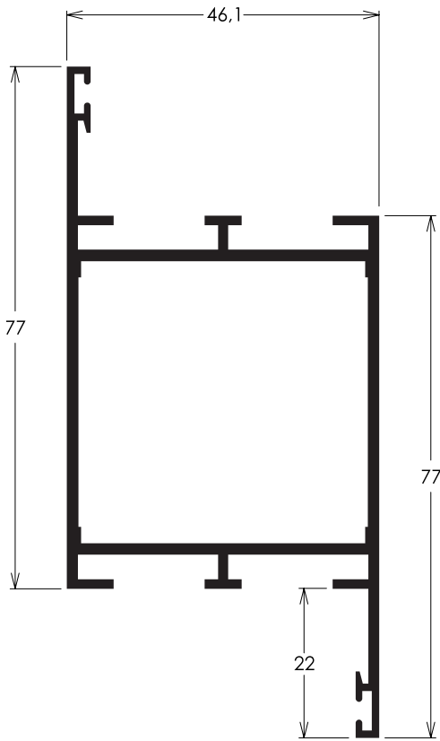
RO042 1,180 kg/m Folha travessa e montante
