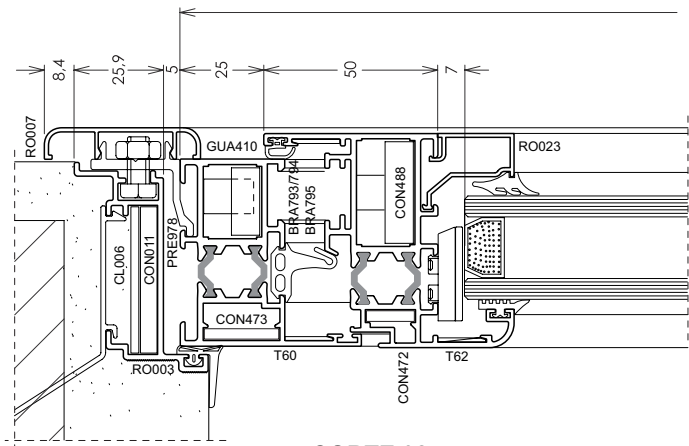
CORTE 02
