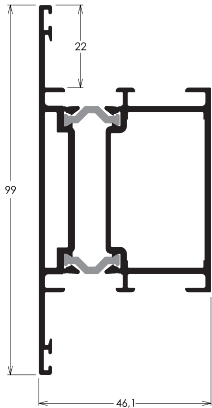
T81 Travessa intermediária
