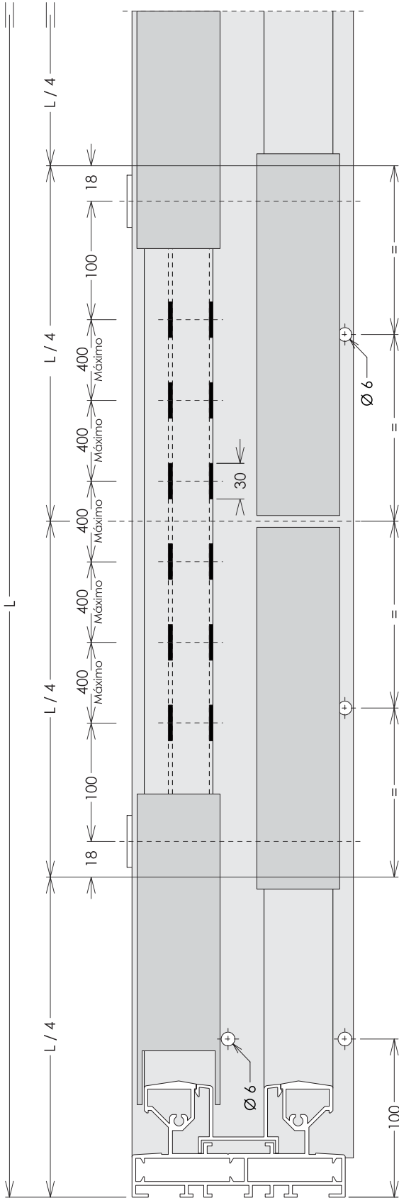
Lado Interno
