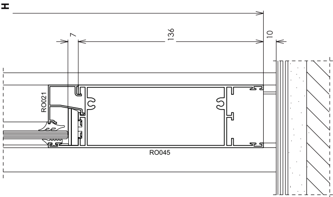
CORTE 01
