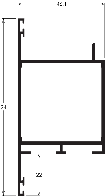
RO043 1,180 kg/m Folha travessa e montante
