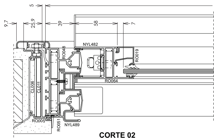
LADO EXTERNO
