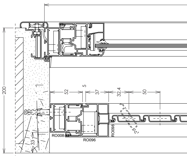
CORTE 02
