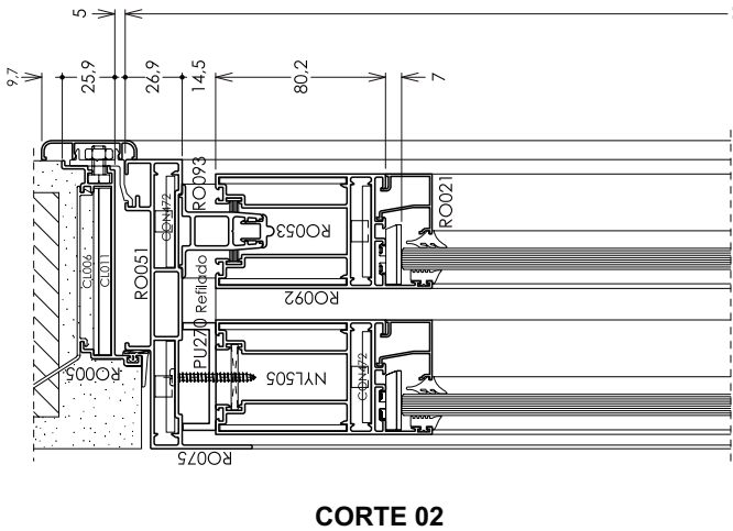
CORTE 02
