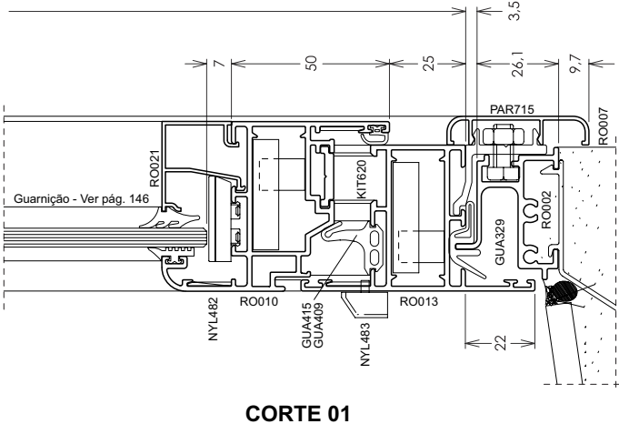
LADO EXTERNO
