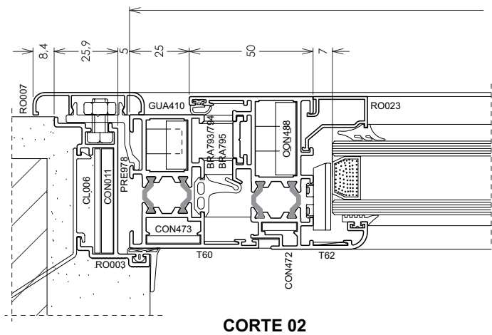
LADO EXTERNO
