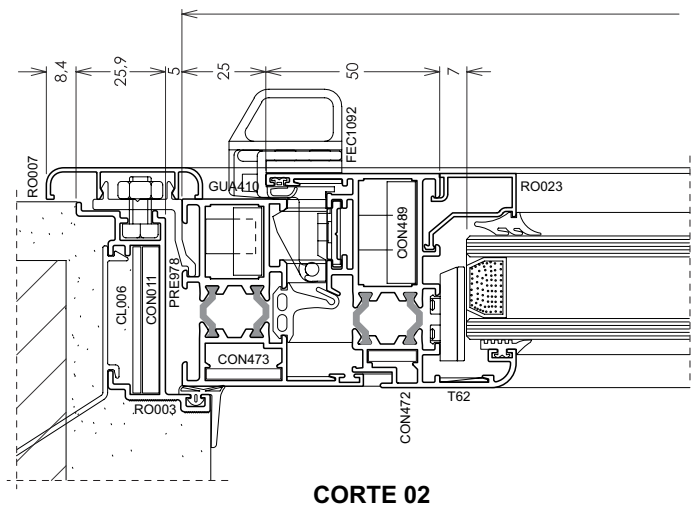
LADO EXTERNO
