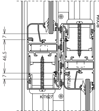
CORTE 04
