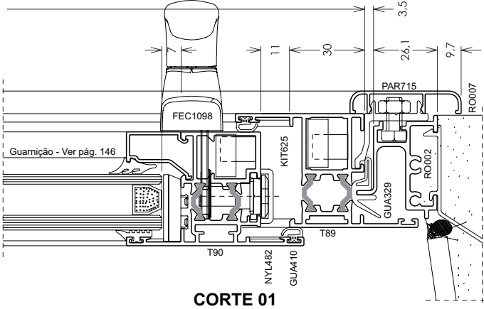
CORTE 01
