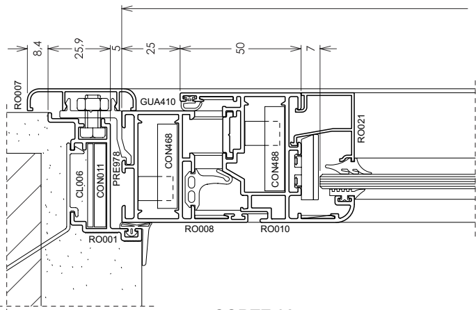
CORTE 02
