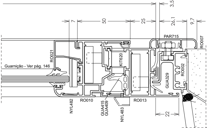
CORTE 01
