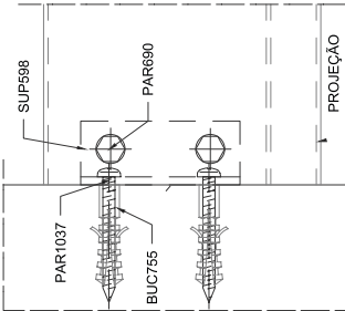
DETALHE - FIXAÇÃO LATERAL VISTA SUPERIOR
