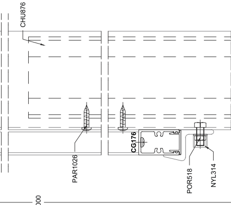
CORTE 01 LADO EXTERNO
