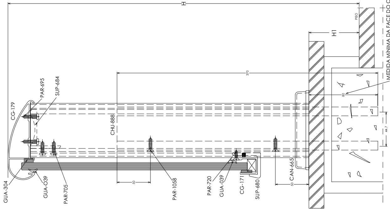
CORTE 01
