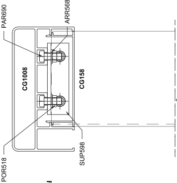
DETALHE - FIXAÇÃO LATERAL CORTE VERTICAL
