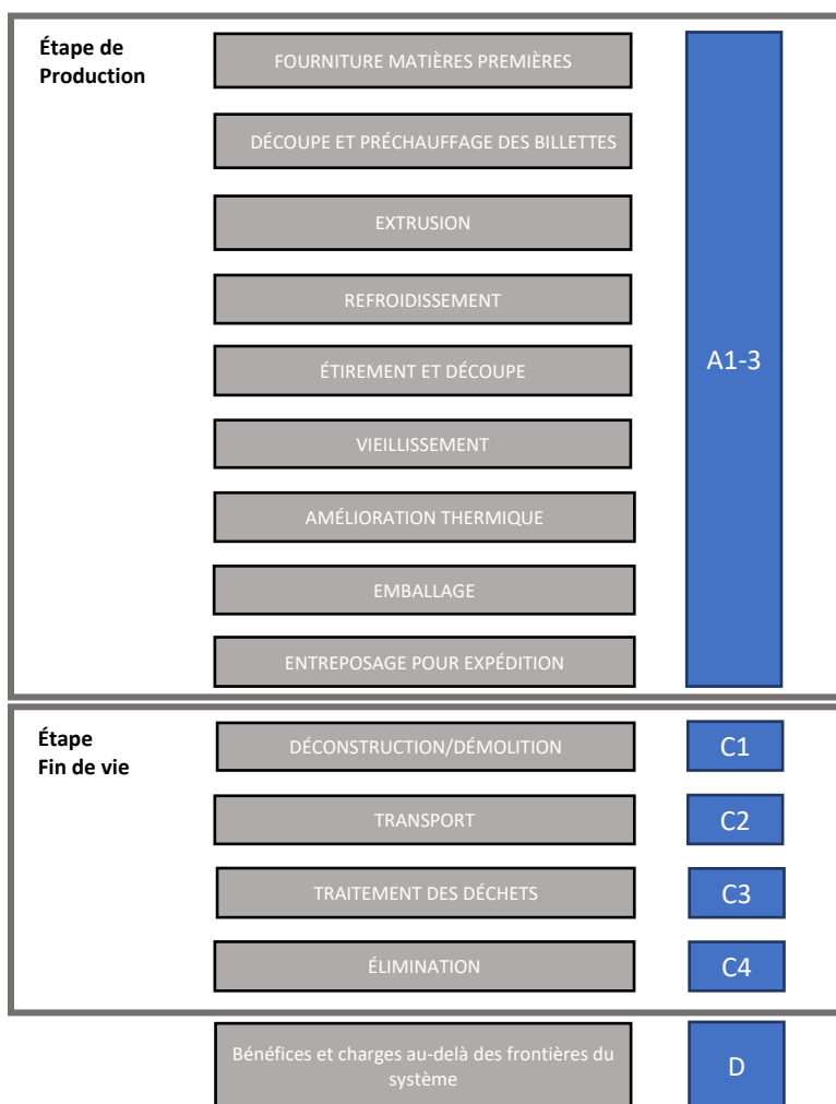
Figure 1 Schéma du processus de fabrication des profilés à Montréal
