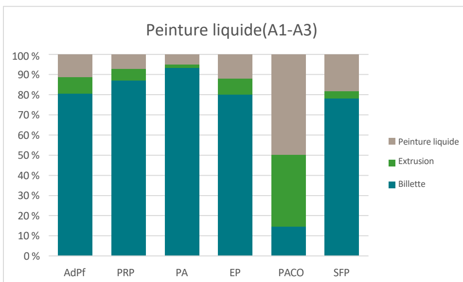
Figure 3 Contribution relative des processus en amont pour le profilé à peinture liquide
