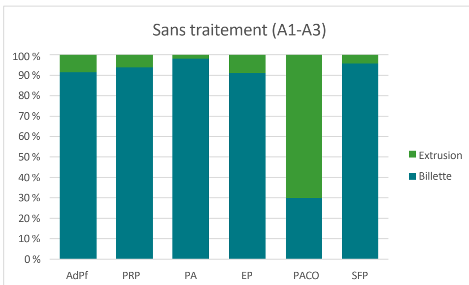
Figure 2 : Contribution relative des processus en amont pour le profilé sans traitement de surface
