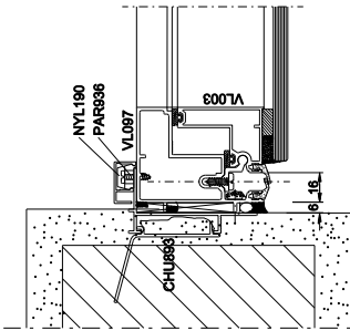
Corte 05 (Opção com perfil VL097)
