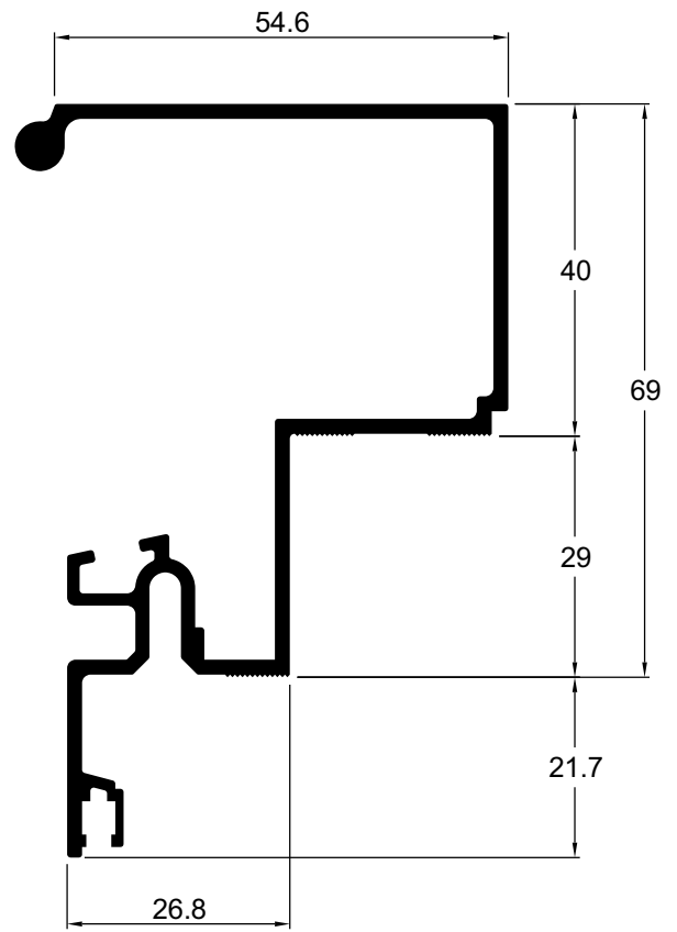
VL036 1,401 kg/m
