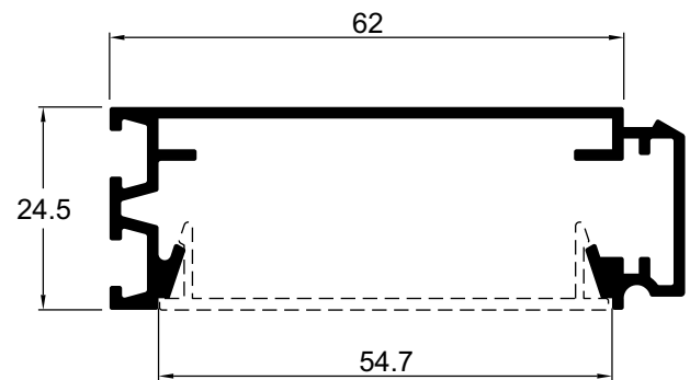
LC036 0,688 kg/m Arremate de folha
