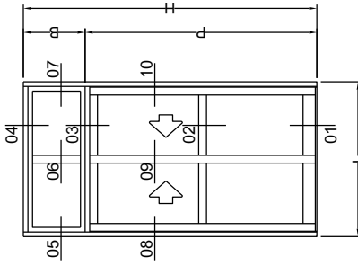
Elevação vista externa
