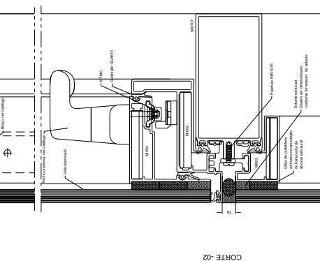
CORTE -02
