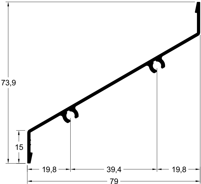
000206 0,602 kg/m Veneziana
