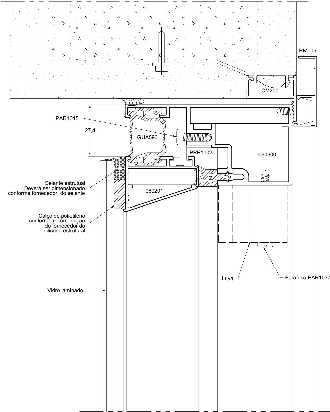
Marco superior com fixo
