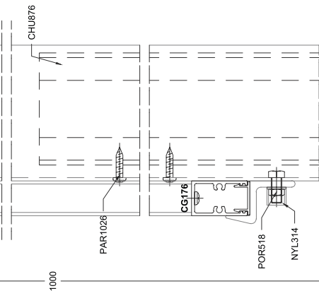
CORTE 01 LADO EXTERNO
