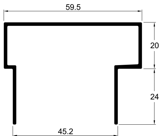
RM043 0,651 Kg/m Tapa da calha
