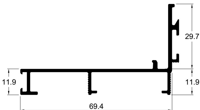
CM234 0,686 Kg/m Contramarco infeior e superior da porta
